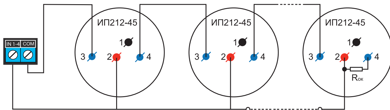
Схема подключения ИП212-45 к пожарному входу NV 2104 только с оконечным резистором
