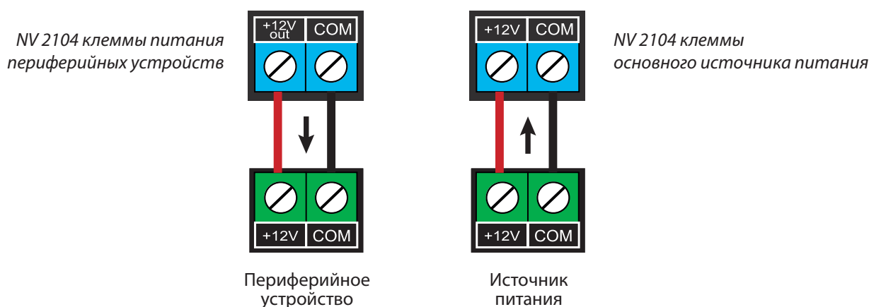
Подключение питания
