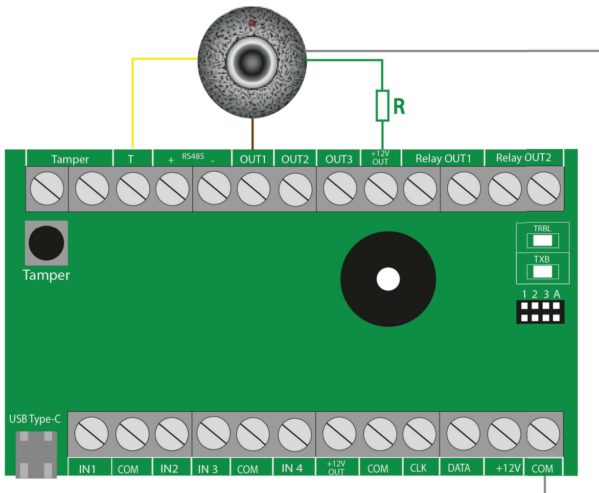
Схема подключения на примере ТМ считывателя СТМ-КТ
